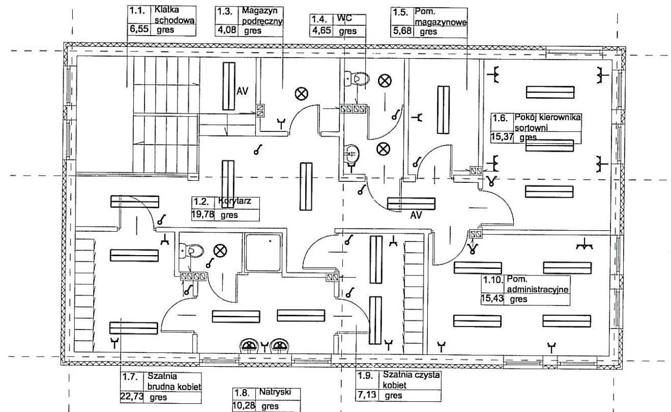
RZUT PIĘTRA
