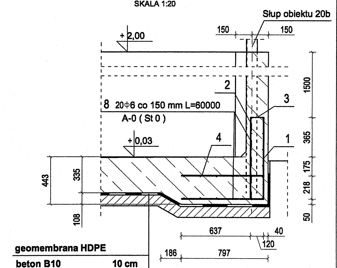
PRZEKRÓJ B1-B1 SKALA 1:20
