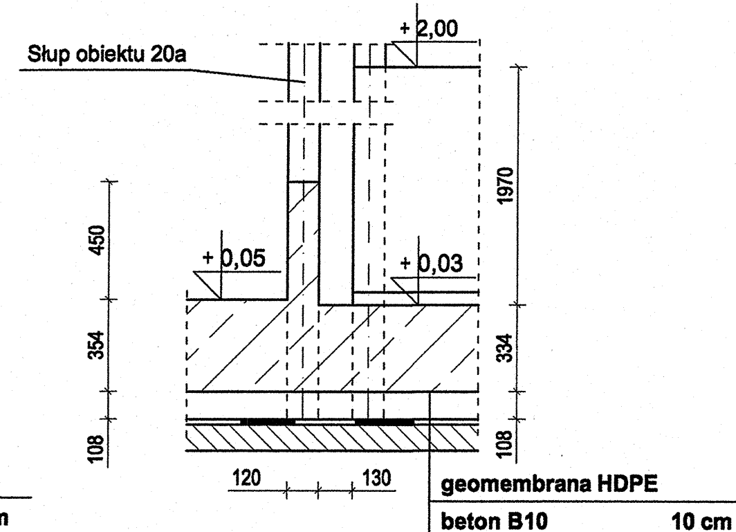
PRZEKRÓJ E-E SKALA 1:20
