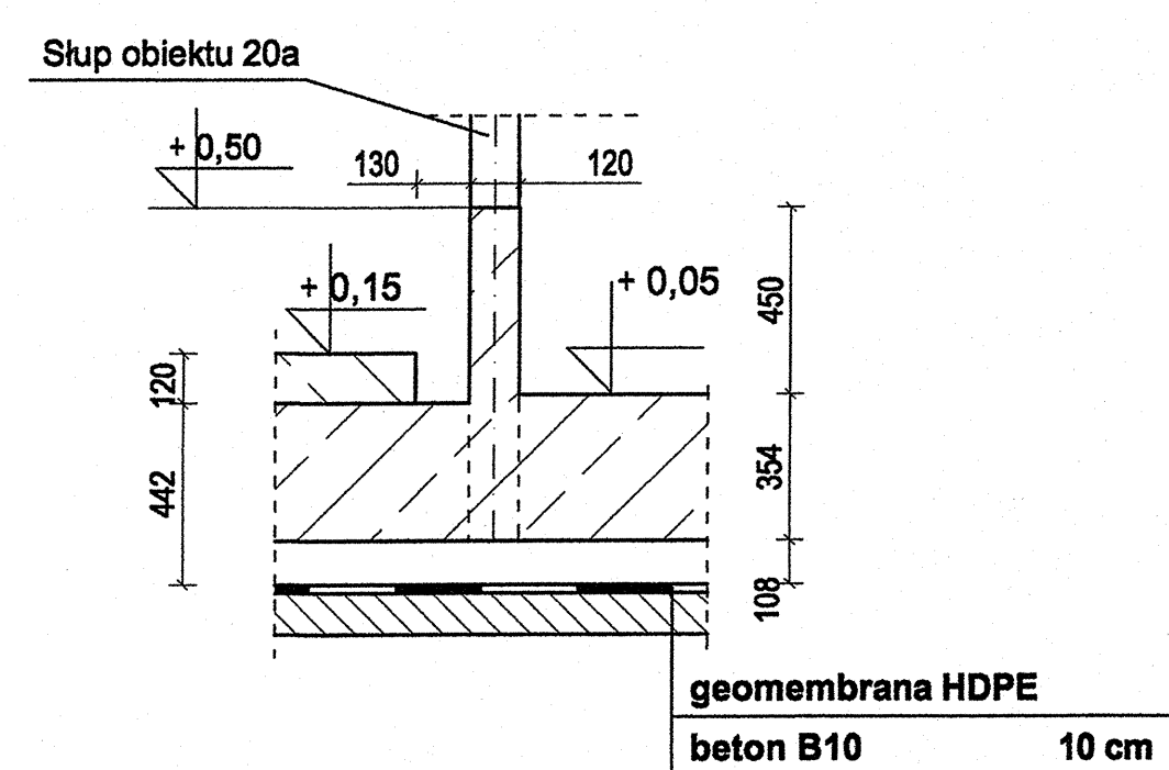
PRZEKRÓJ D-D SKALA 1:20
