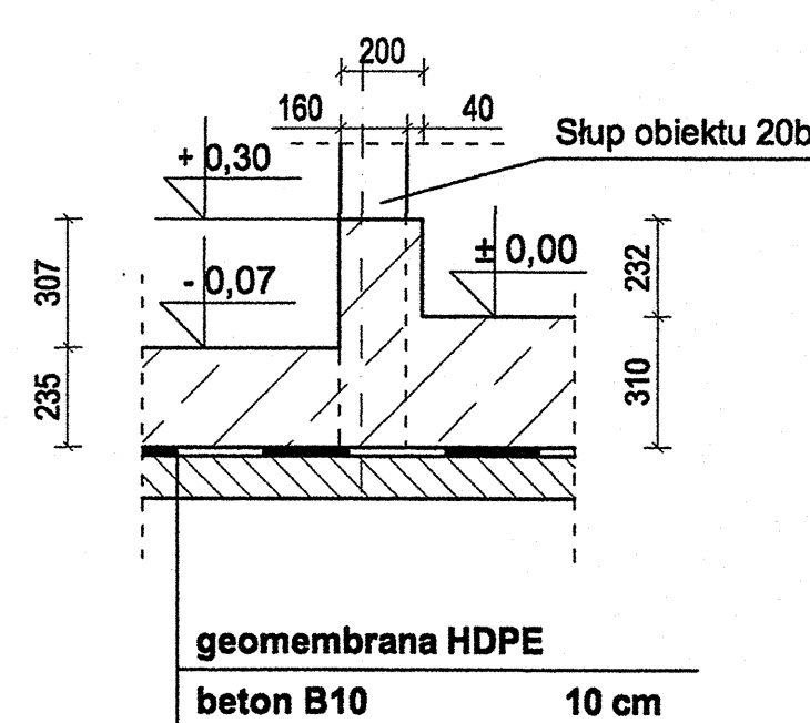
PRZEKRÓJ G-G SKALA 1:20
