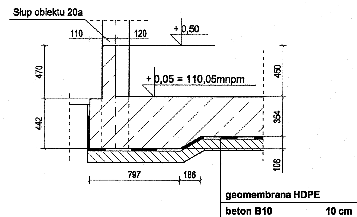
PRZEKRÓJ G-G SKALA 1:20
