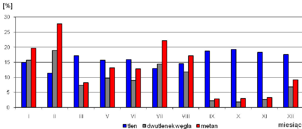
Ryc. 2. Zmienność procentowej zawartości O 2 , CO 2 i CH 4 w gazie składowiskowym w punkcie S-2
