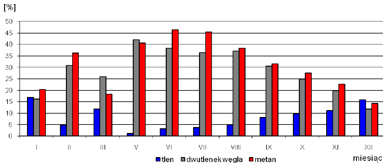
Ryc. 3. Zmienność procentowej zawartości O 2 , CO 2 i CH 4 w gazie składowiskowym w punkcie S-3
