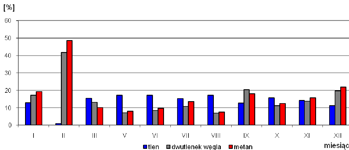
Ryc. 1. Zmienność procentowej zawartości O 2 , CO 2 i CH 4 w gazie składowiskowym w punkcie S-1
